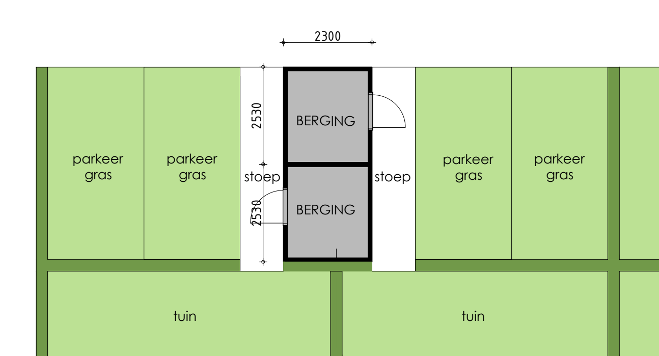
Plattegrond
