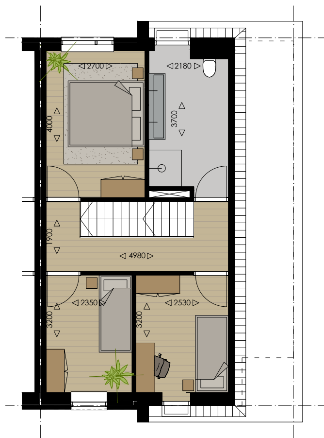
1e verdieping
