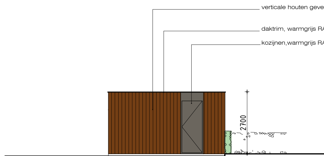
Zijgevel
