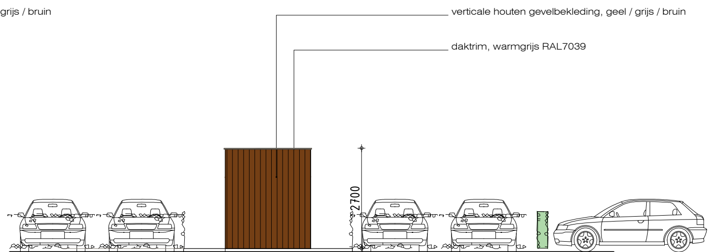
Kopgevel
